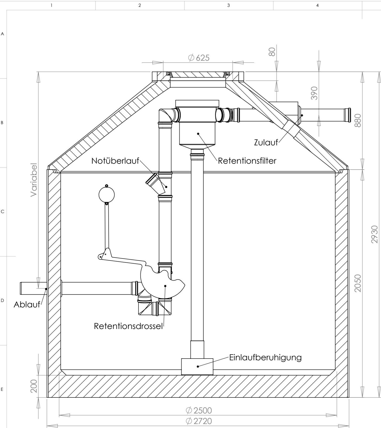
SCHNITT A-A
