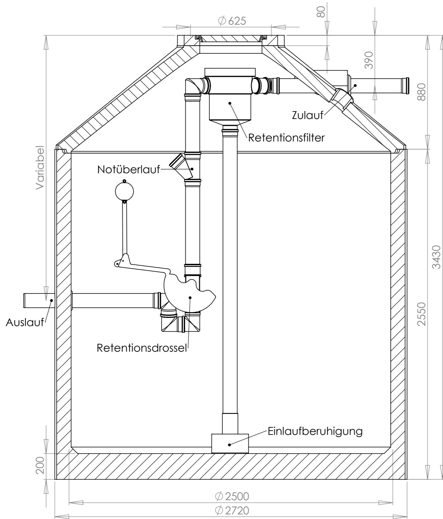
SCHNITT A-A
