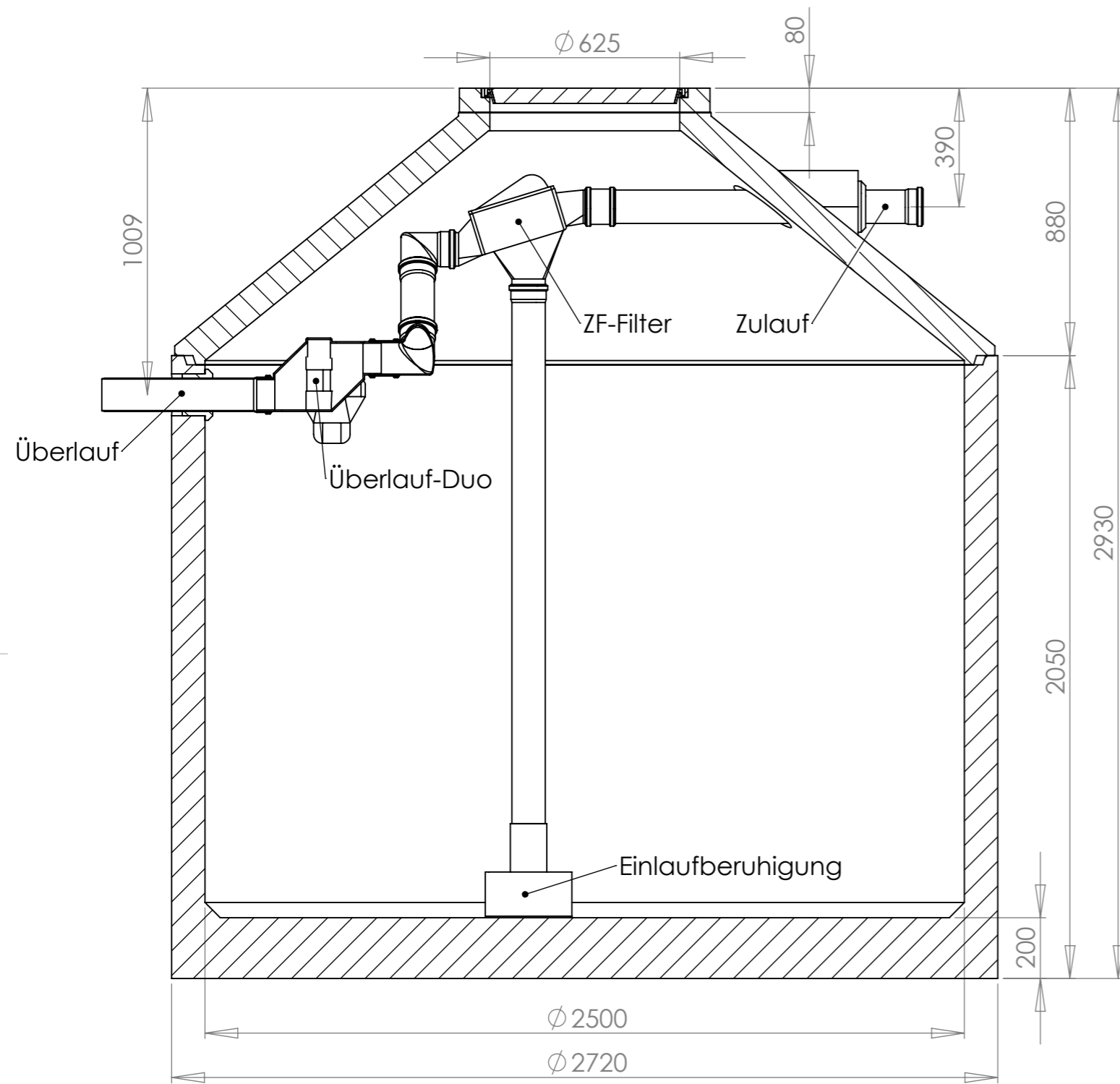
SCHNITT A-A
