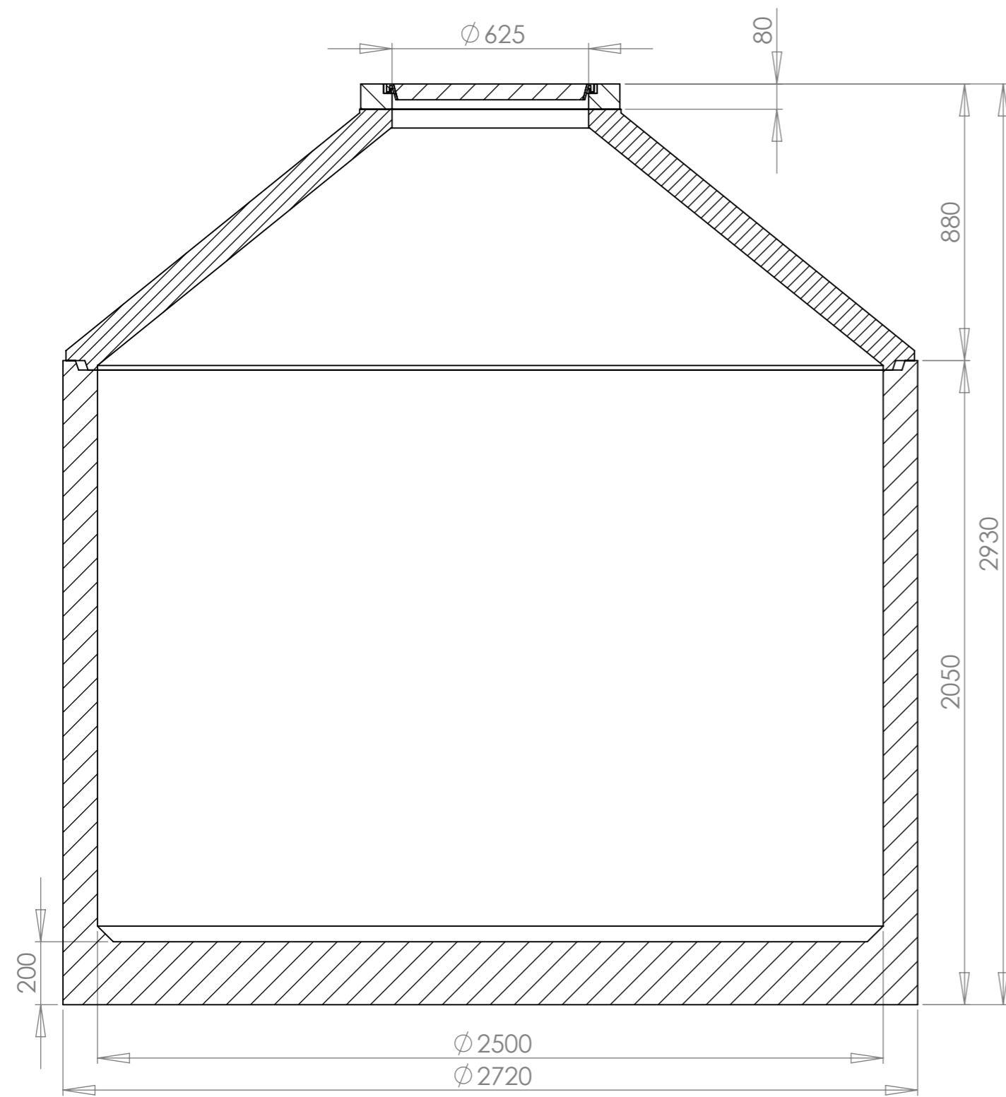
SCHNITT A-A
