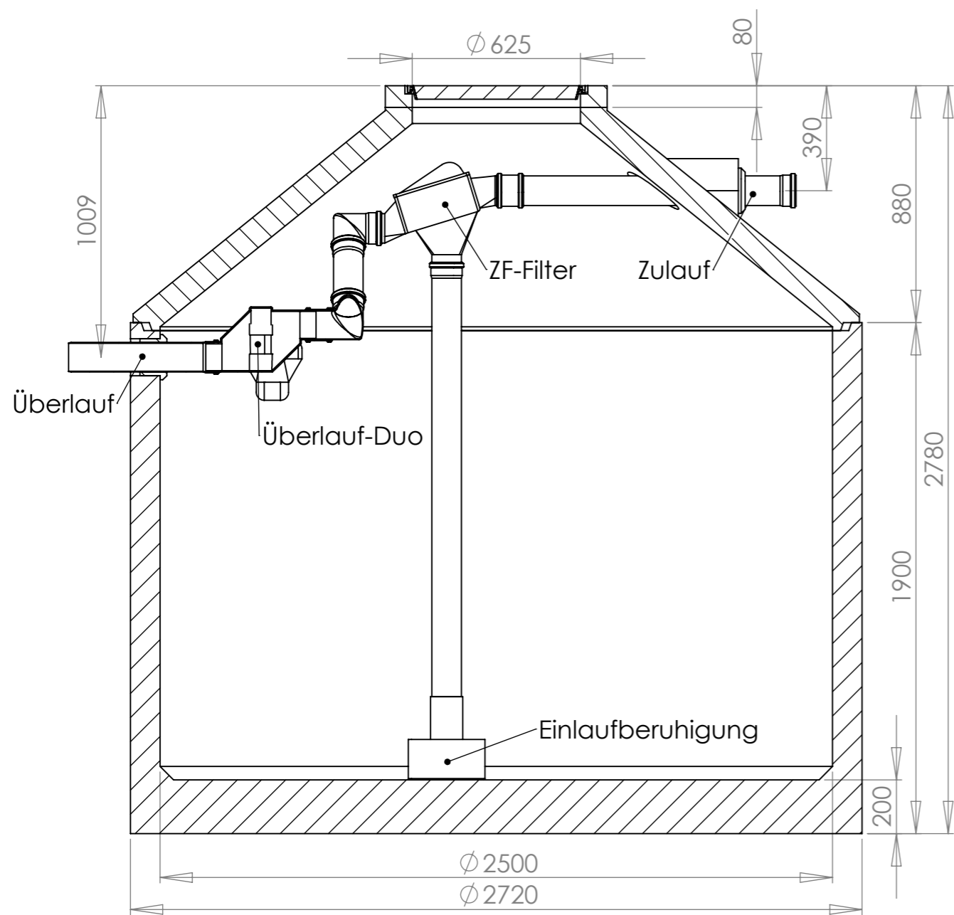
SCHNITT A-A
