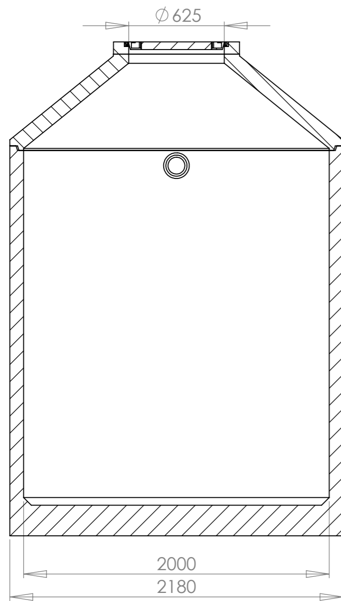
SCHNITT B-B
