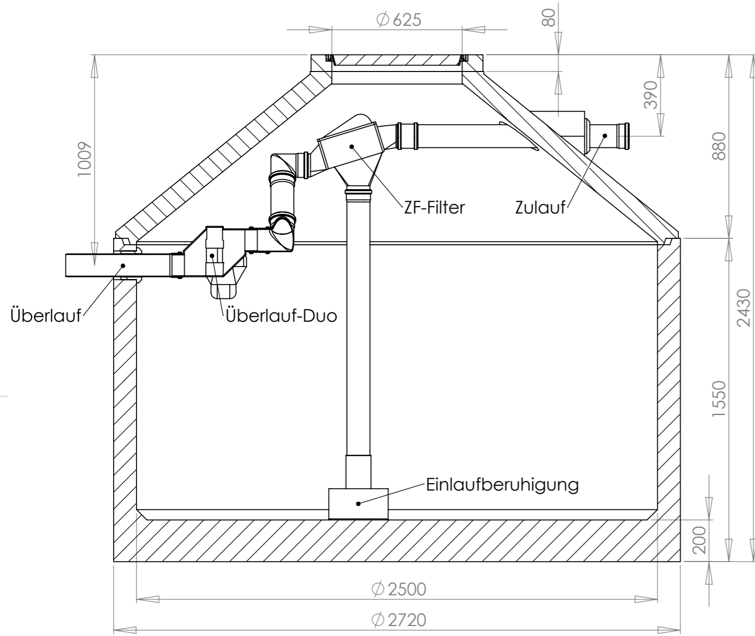
SCHNITT A-A
