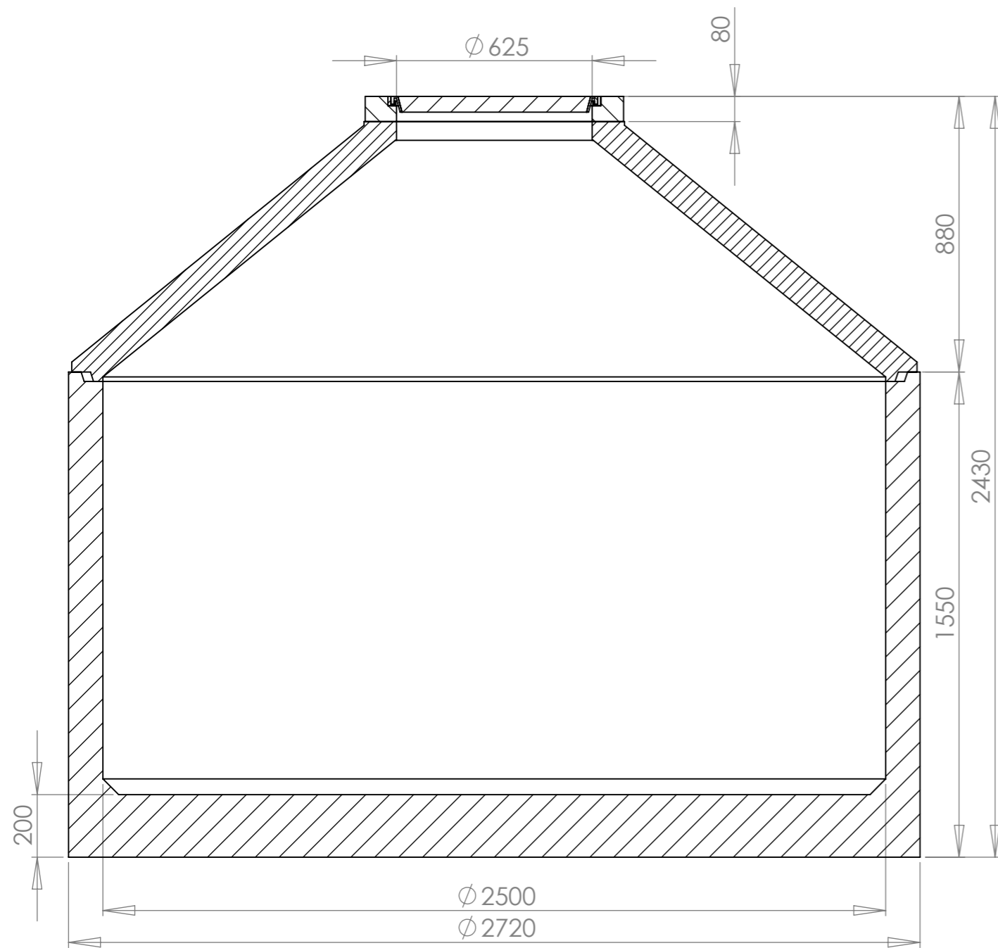
SCHNITT A-A
