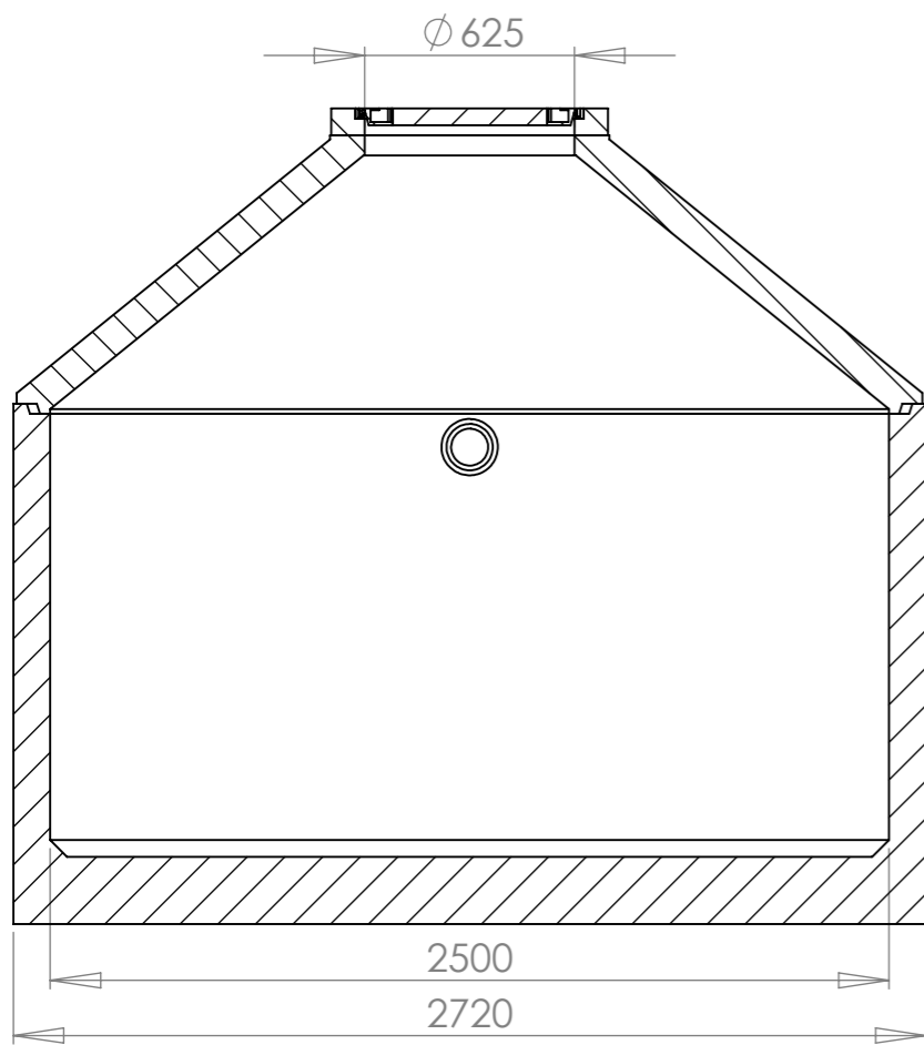
SCHNITT B-B
