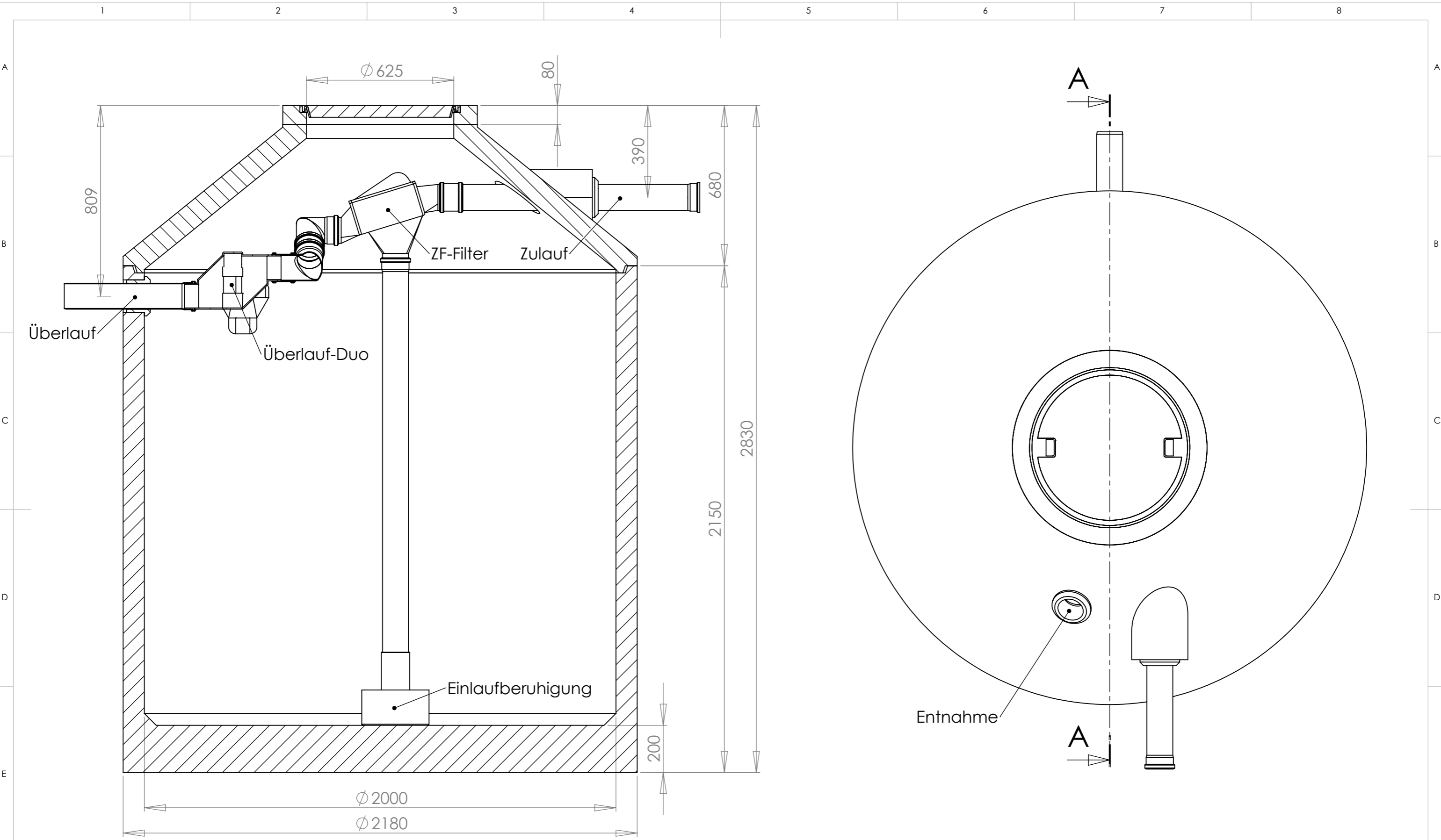
SCHNITT A-A
