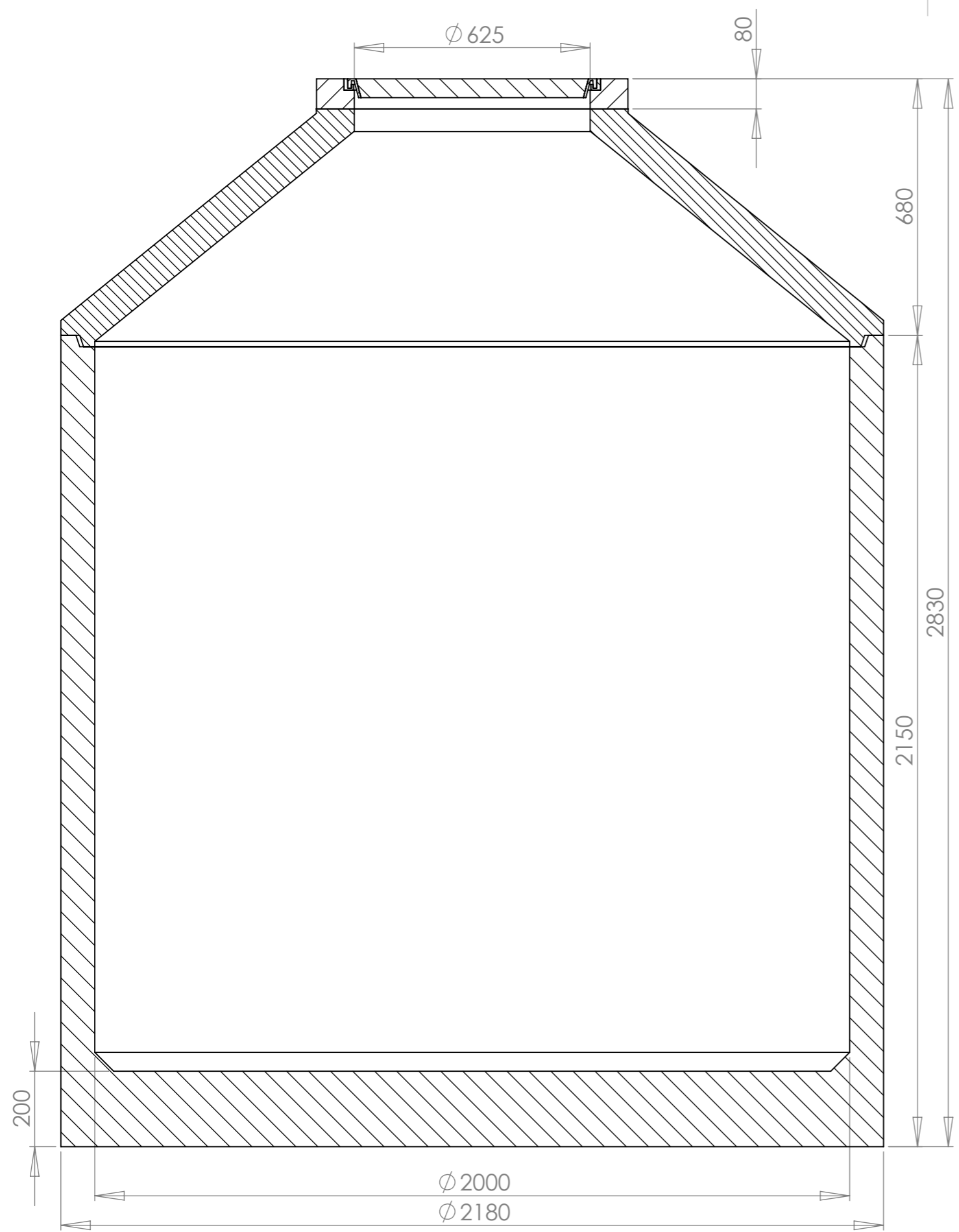
SCHNITT A-A
