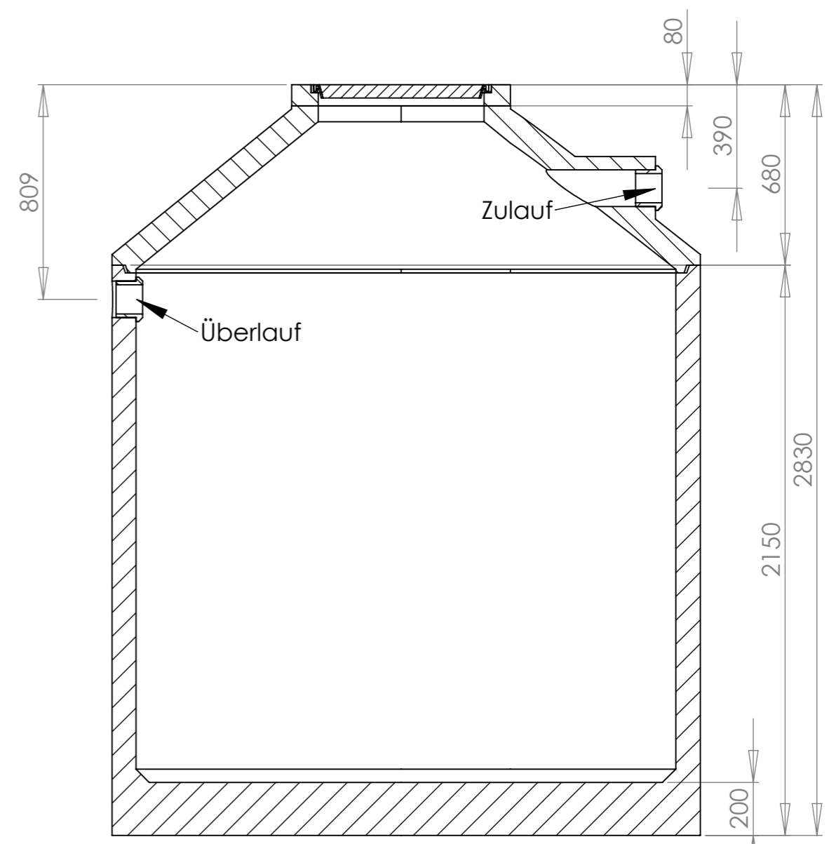
SCHNITT A-A
