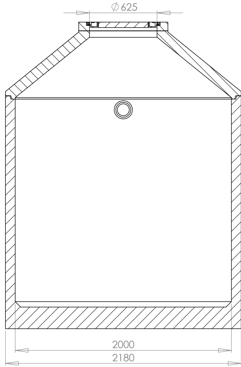
SCHNITT B-B
