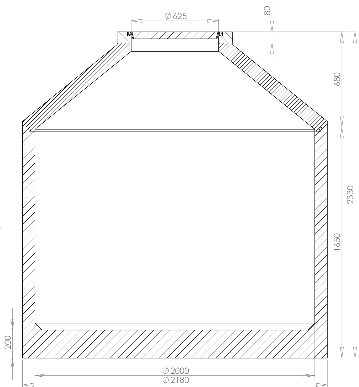
SCHNITT A-A
