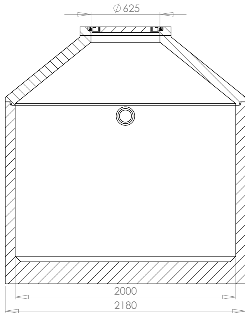
SCHNITT B-B
