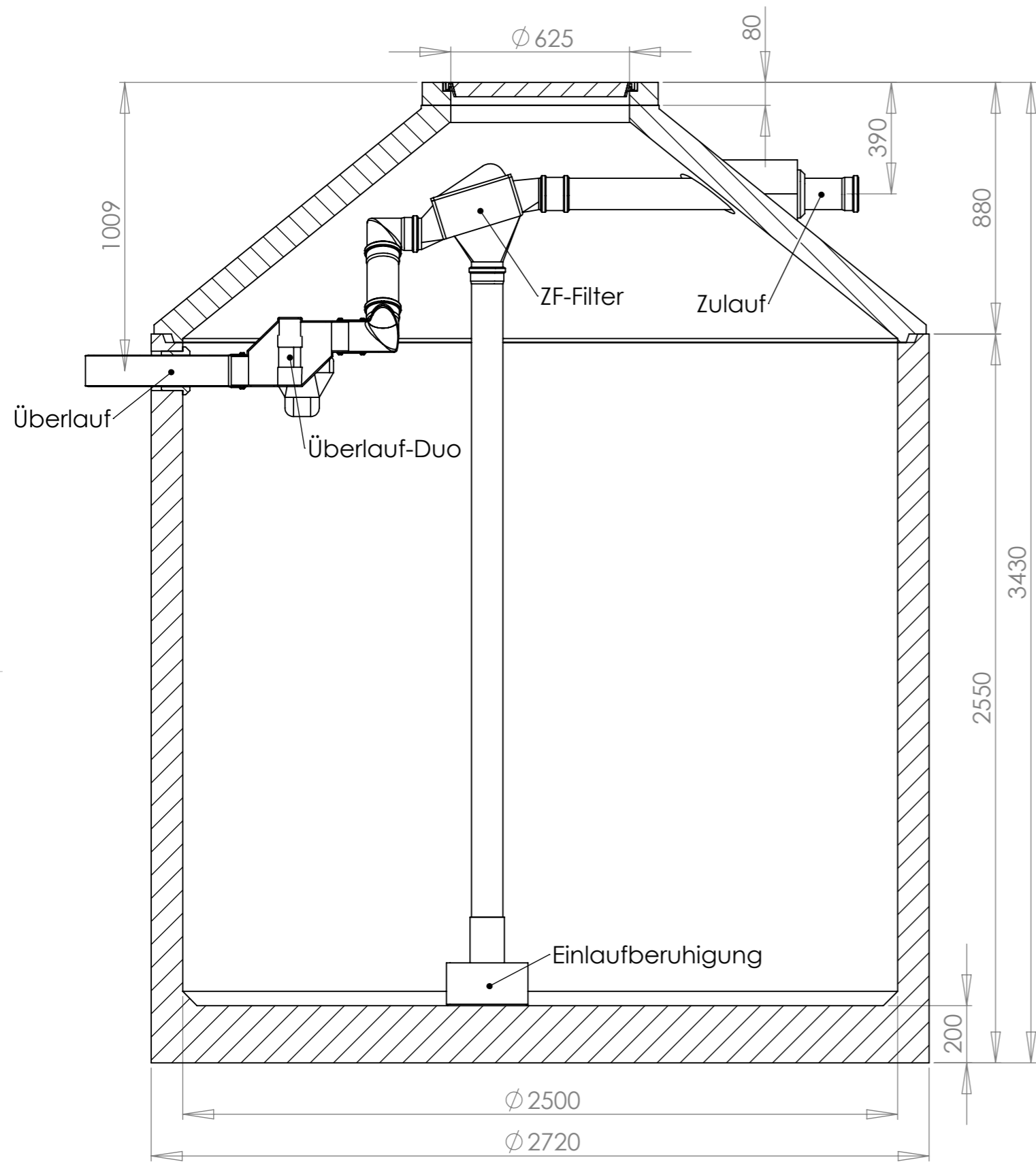
SCHNITT A-A
