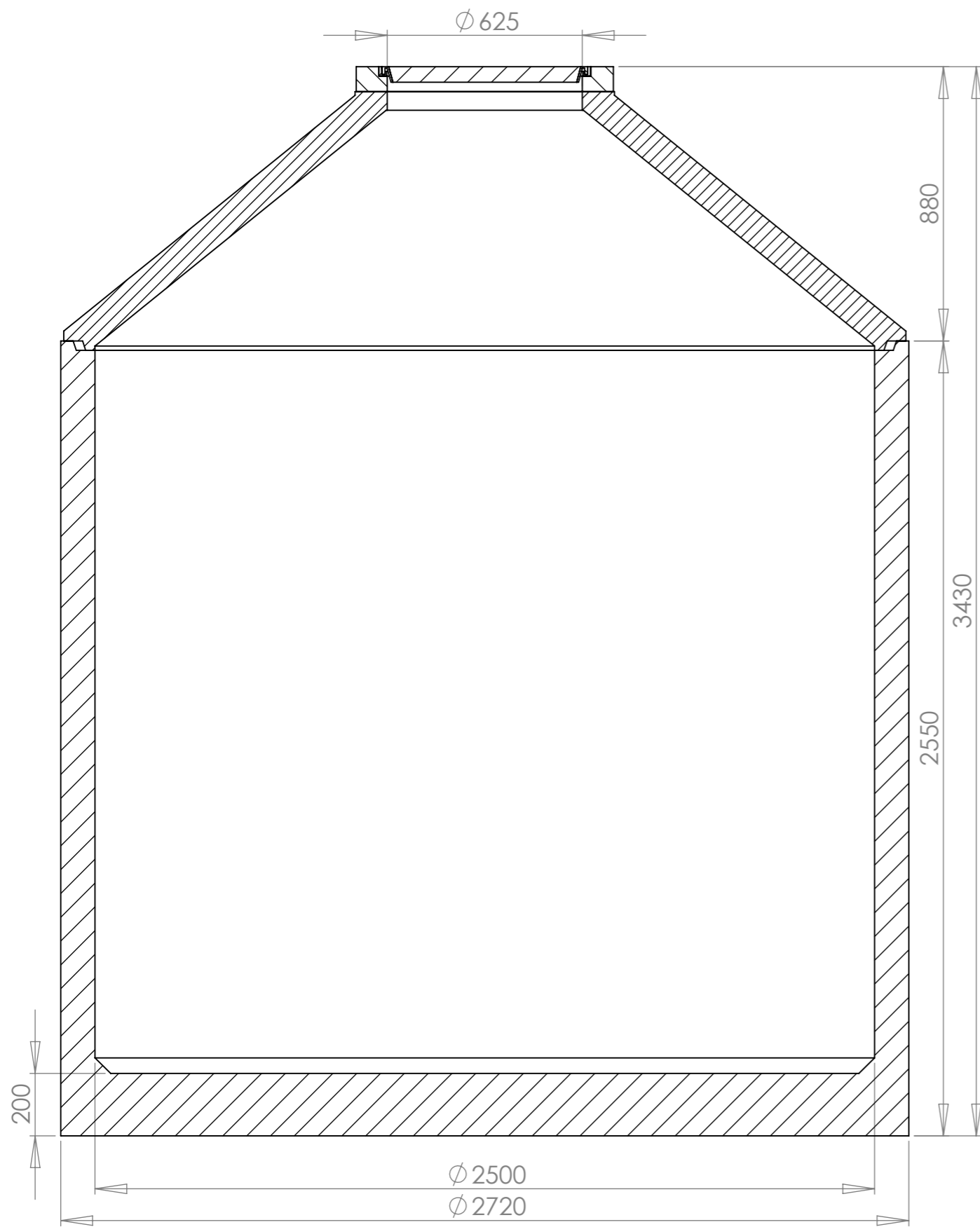
SCHNITT A-A
