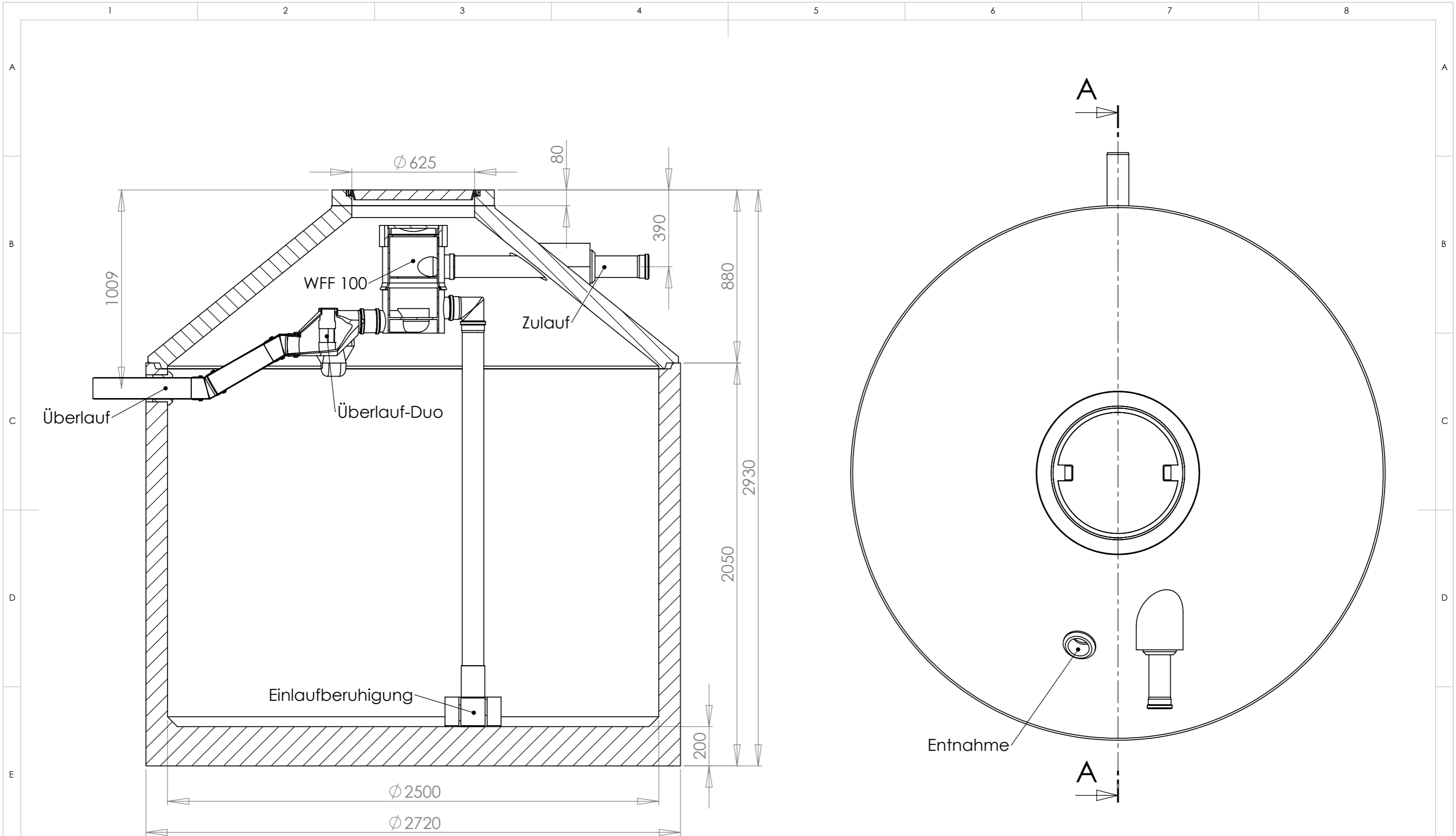
SCHNITT A-A
