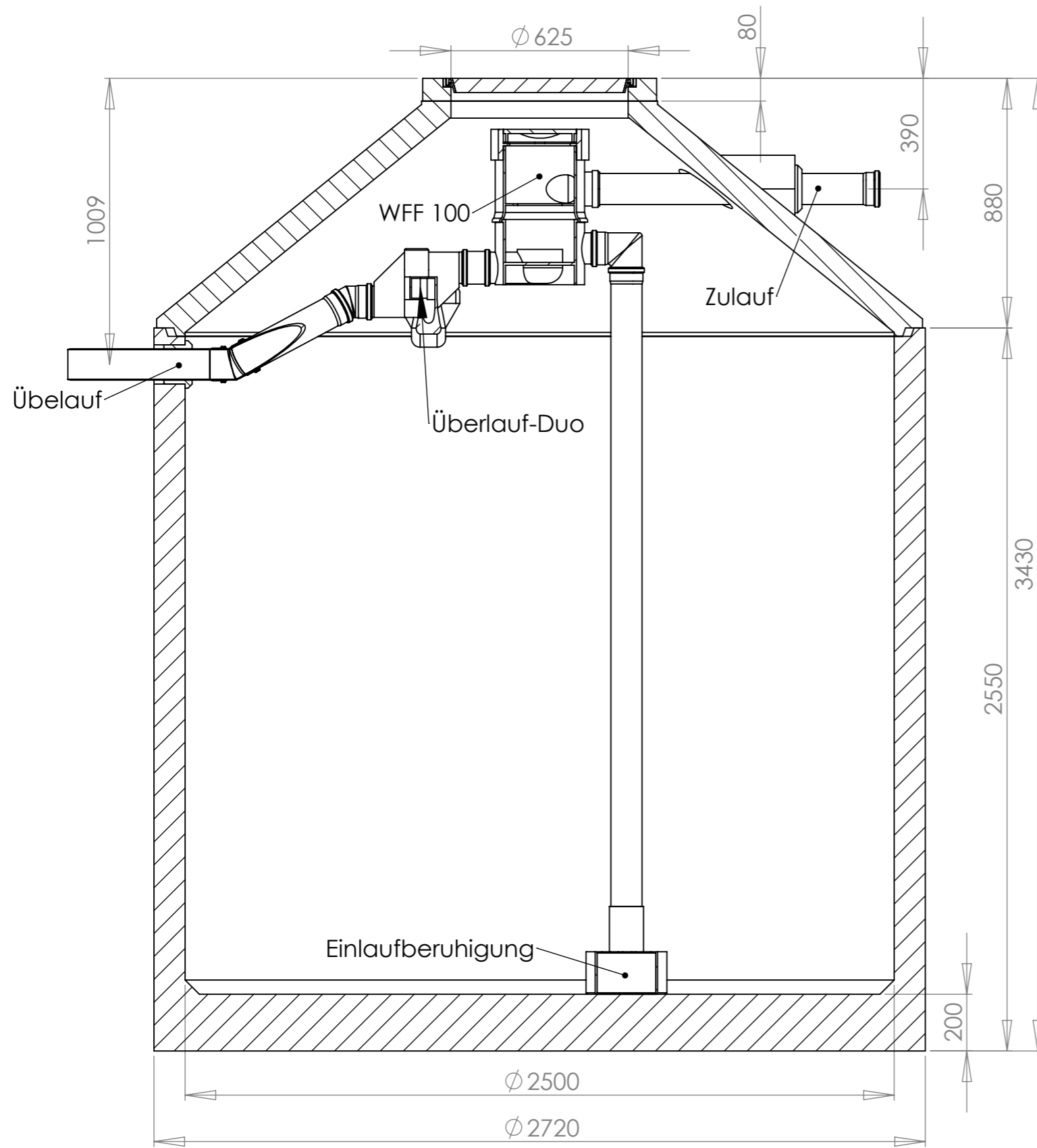
SCHNITT A-A
