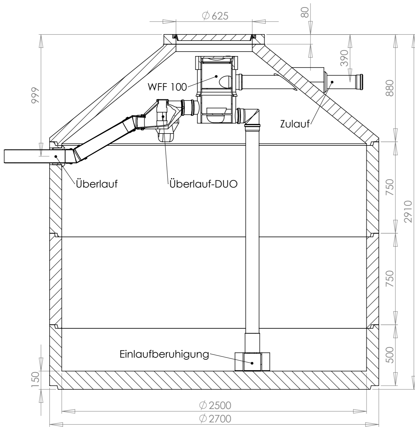
SCHNITT A-A
