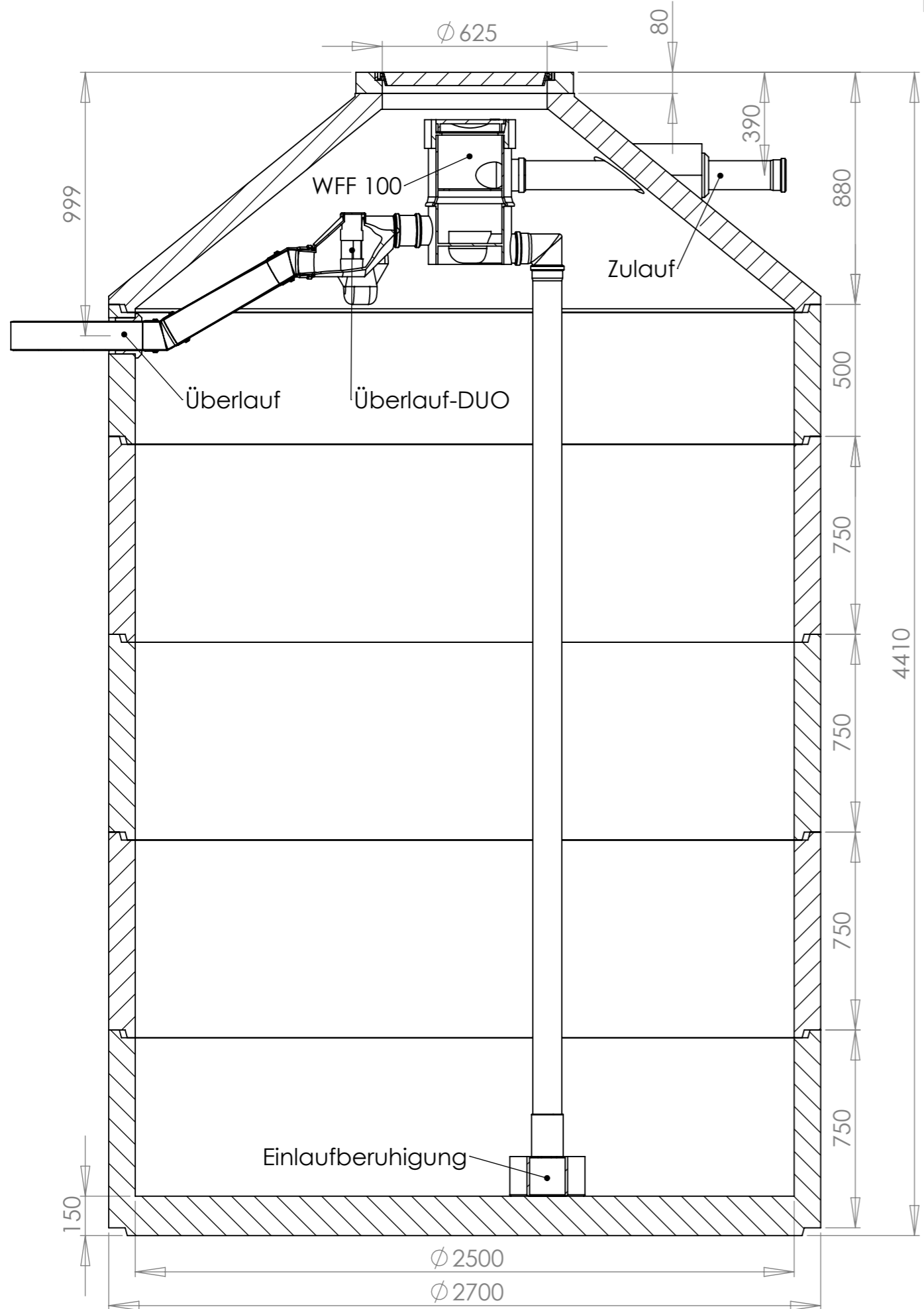
SCHNITT A-A
