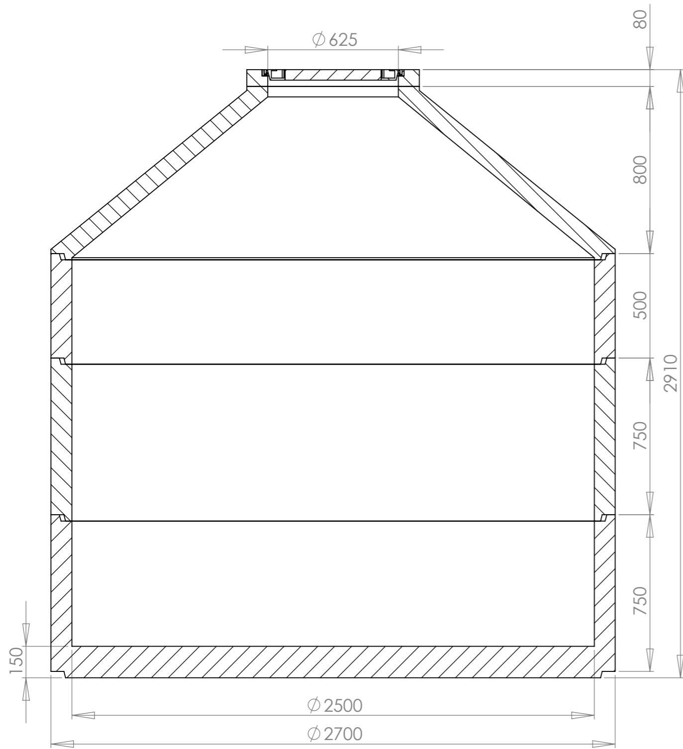
SCHNITT A-A
