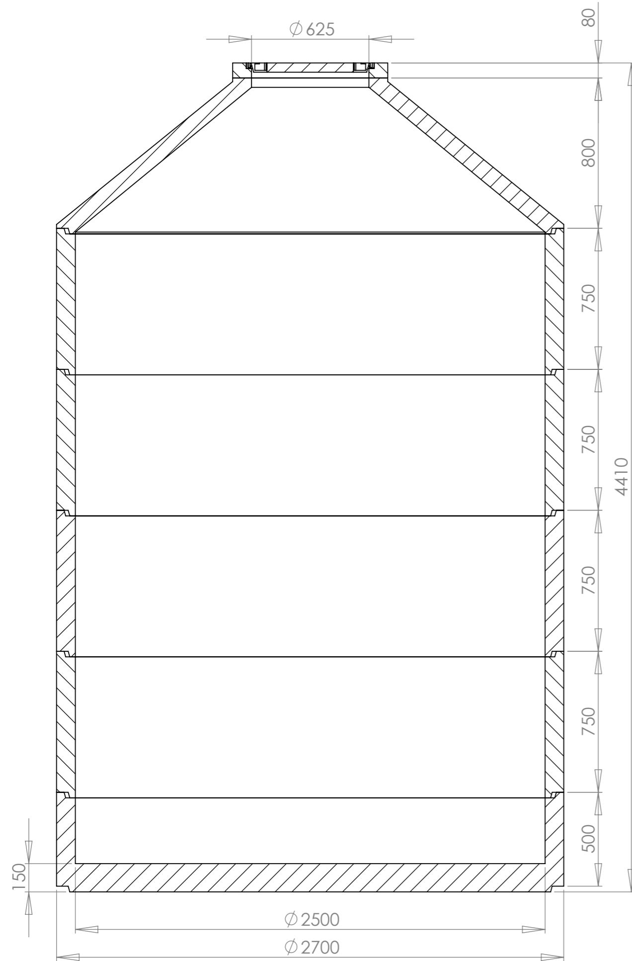
SCHNITT A-A
